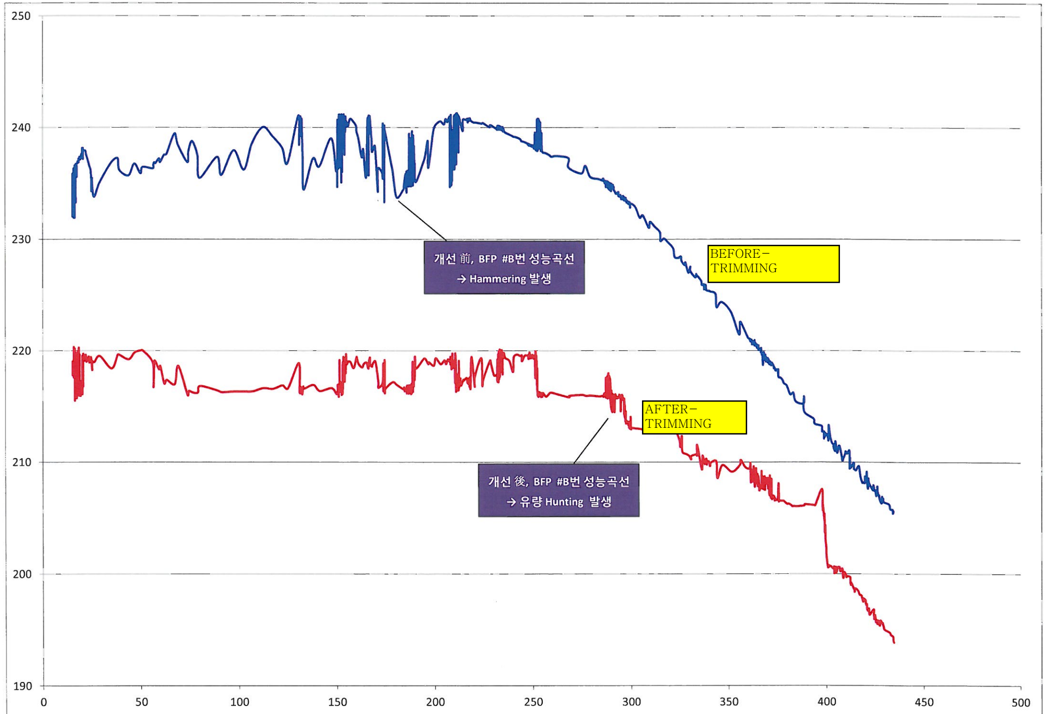
2015년 11월 6일 15:00 시 보일러 급수펌프 #B TEST 결과
