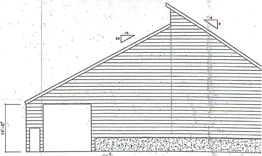
LEFT ENDWALL ELEVATION SCALE: 1/8" = 1'-0"
