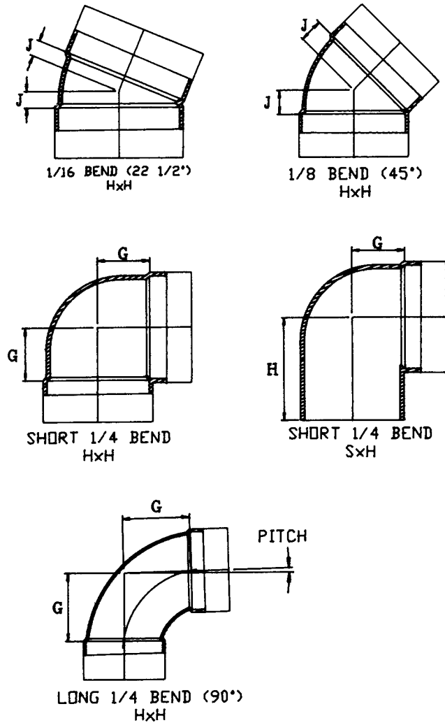
FIG. X3.1 Bends
