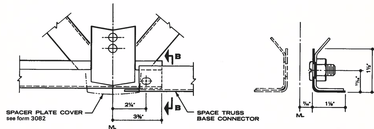
DETAIL A Scale: 3"=1'-0"
