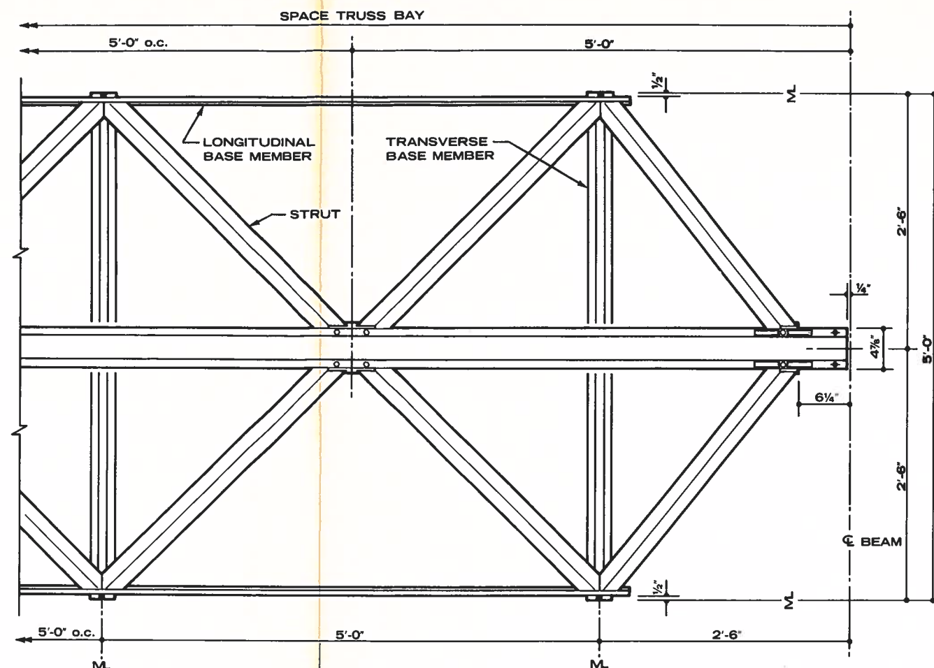
PLAN Scale: 1/8"=1'-0"
