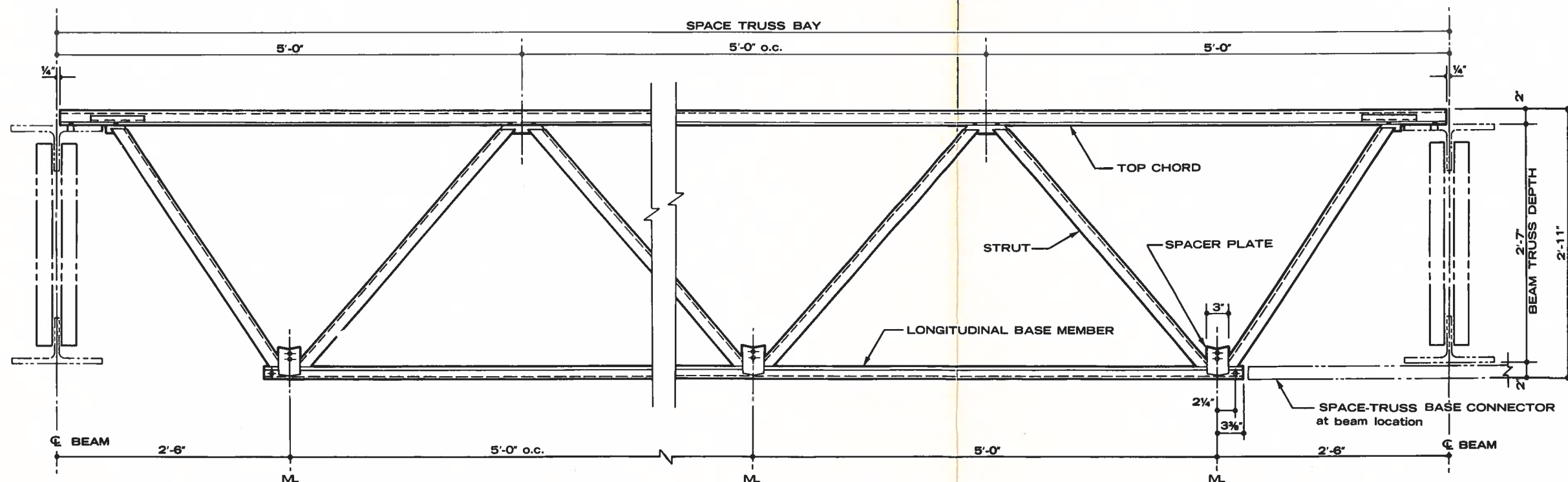
ELEVATION Scale: 1/8"=1'-0"
