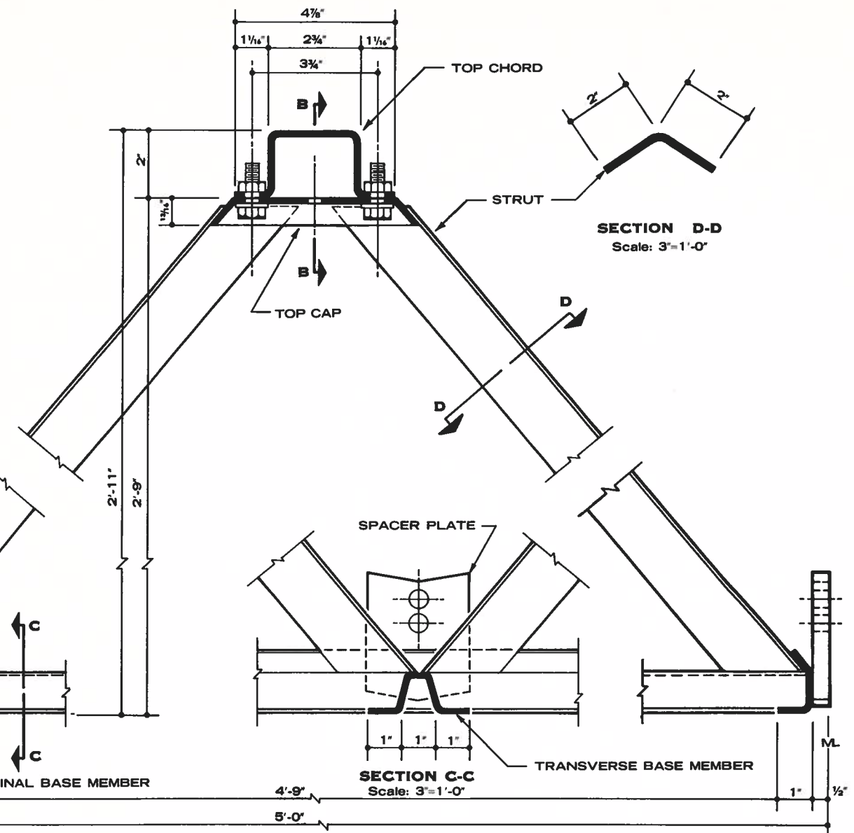
SECTION THRU SPACE TRUSS Scale: 3"=1'-0"
