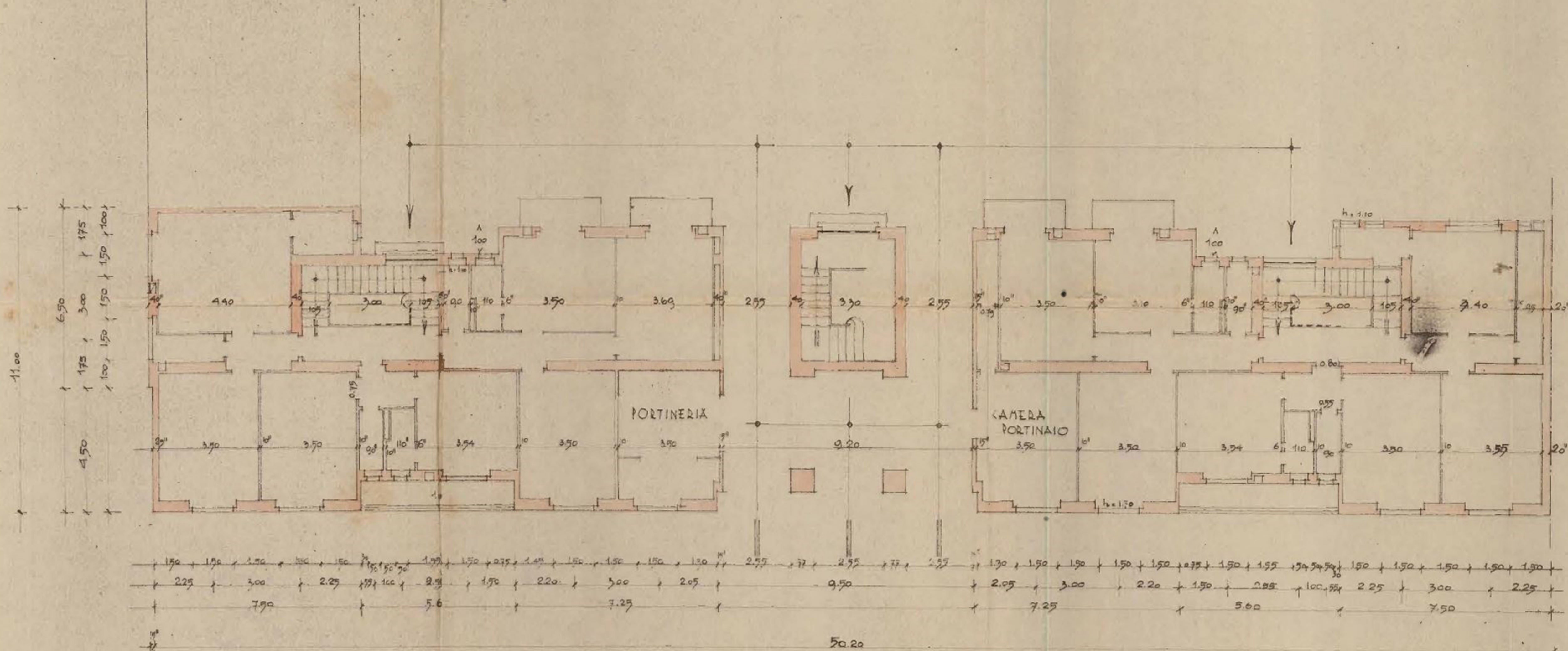
FABBRICATO 1 PIANTA PIANO TERRENO RAPP. 1:100
