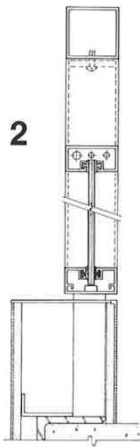
ELEVATION
