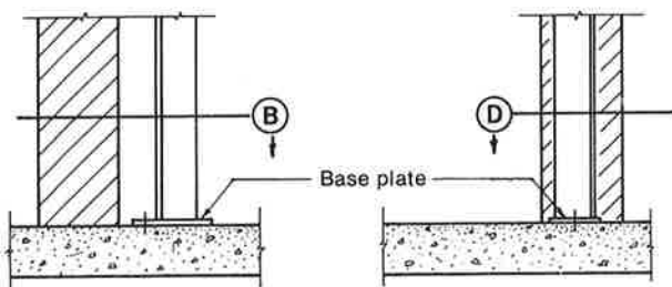
ELEVATION
