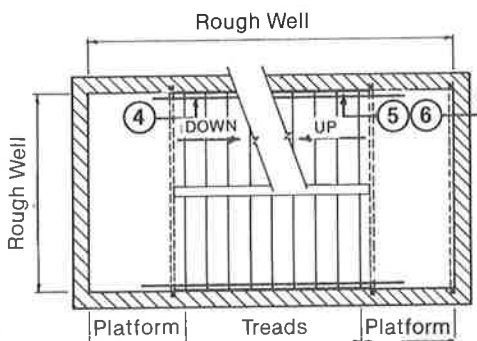
PLAN A-A
