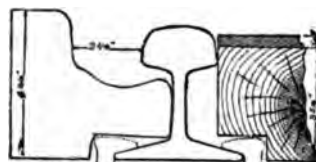
Section on E F.
