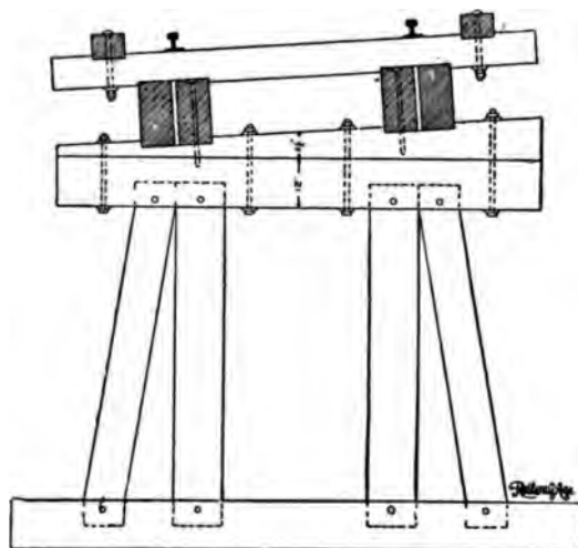
FIG. 124B.—CUSHION CAP.
