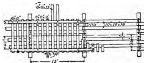
FIG. 3.—FLOOR-SYSTEM.
