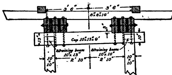
FIG. 125.—NOTCHING CAP.
