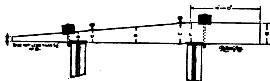
FIG. 123A.—TAPERED TIE.
