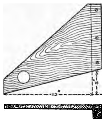
FIG. 45. BATTER-POST TEMPLATE.
