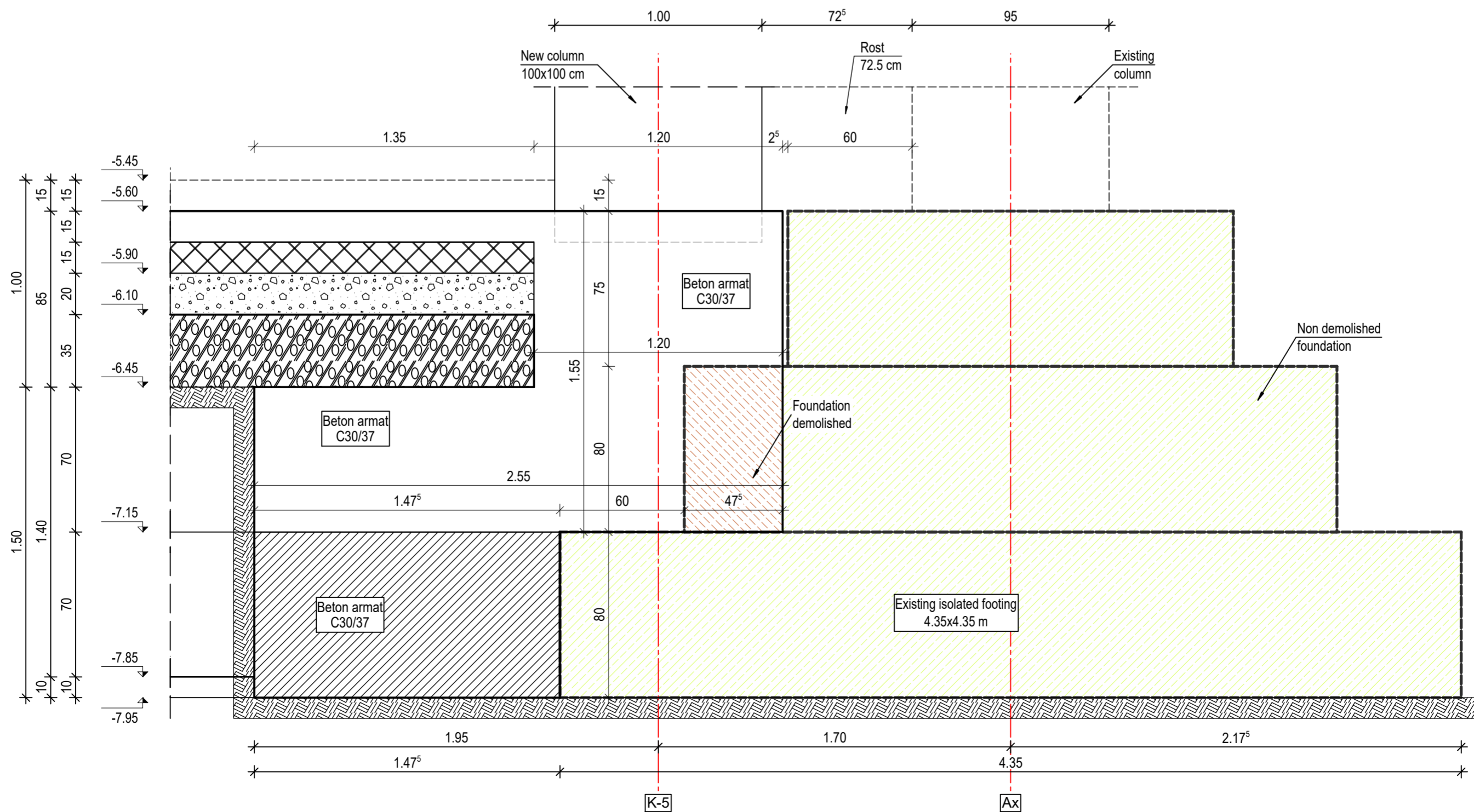
Sectiune E - E Scara 1:20
