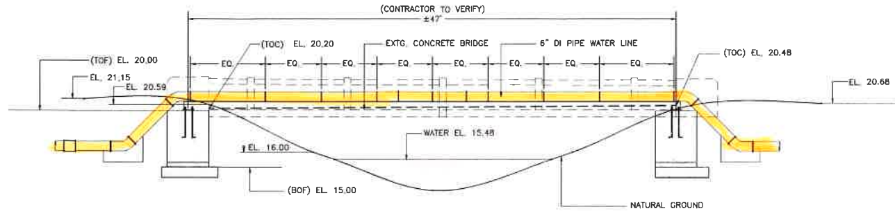
2 ELEVATION C-C SCALE: 1/4"=1'-0"
