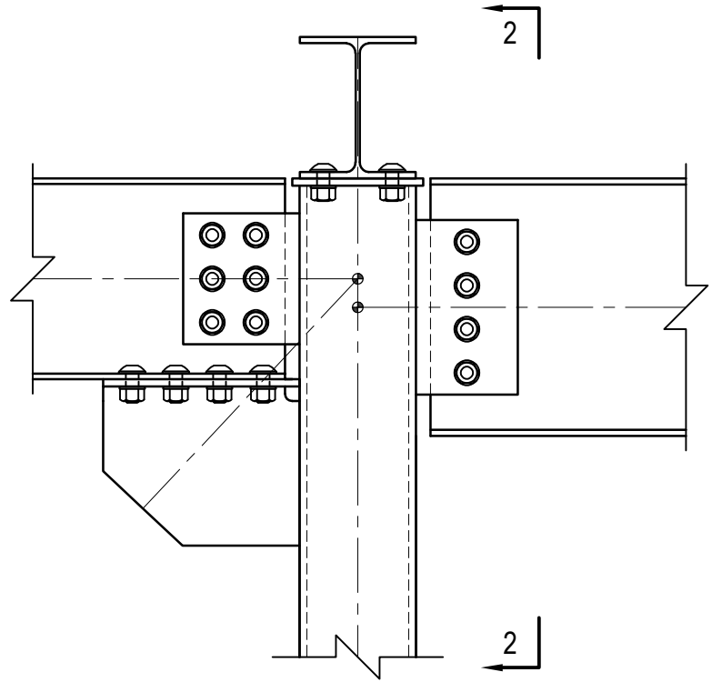
DETAIL A-ALT
